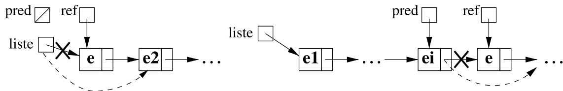
FIGURE 14.3 – Suppression d'une cellule de la liste
