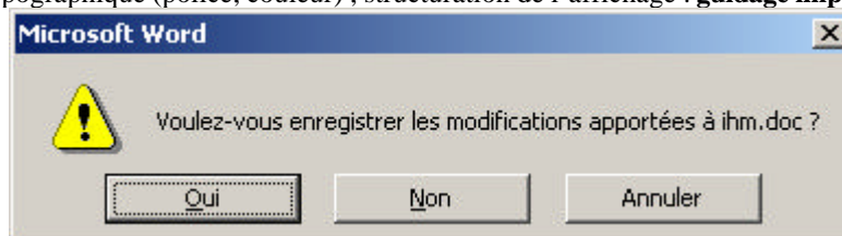
fig 2 : Message d'avertissement
