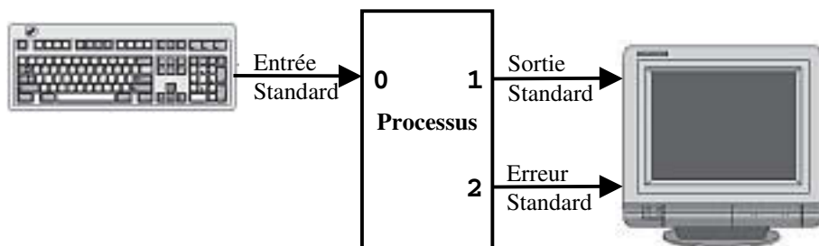
FIGURE 7.1. ENTRÉES/SORTIES STANDARD D'UN PROCESSUS.
