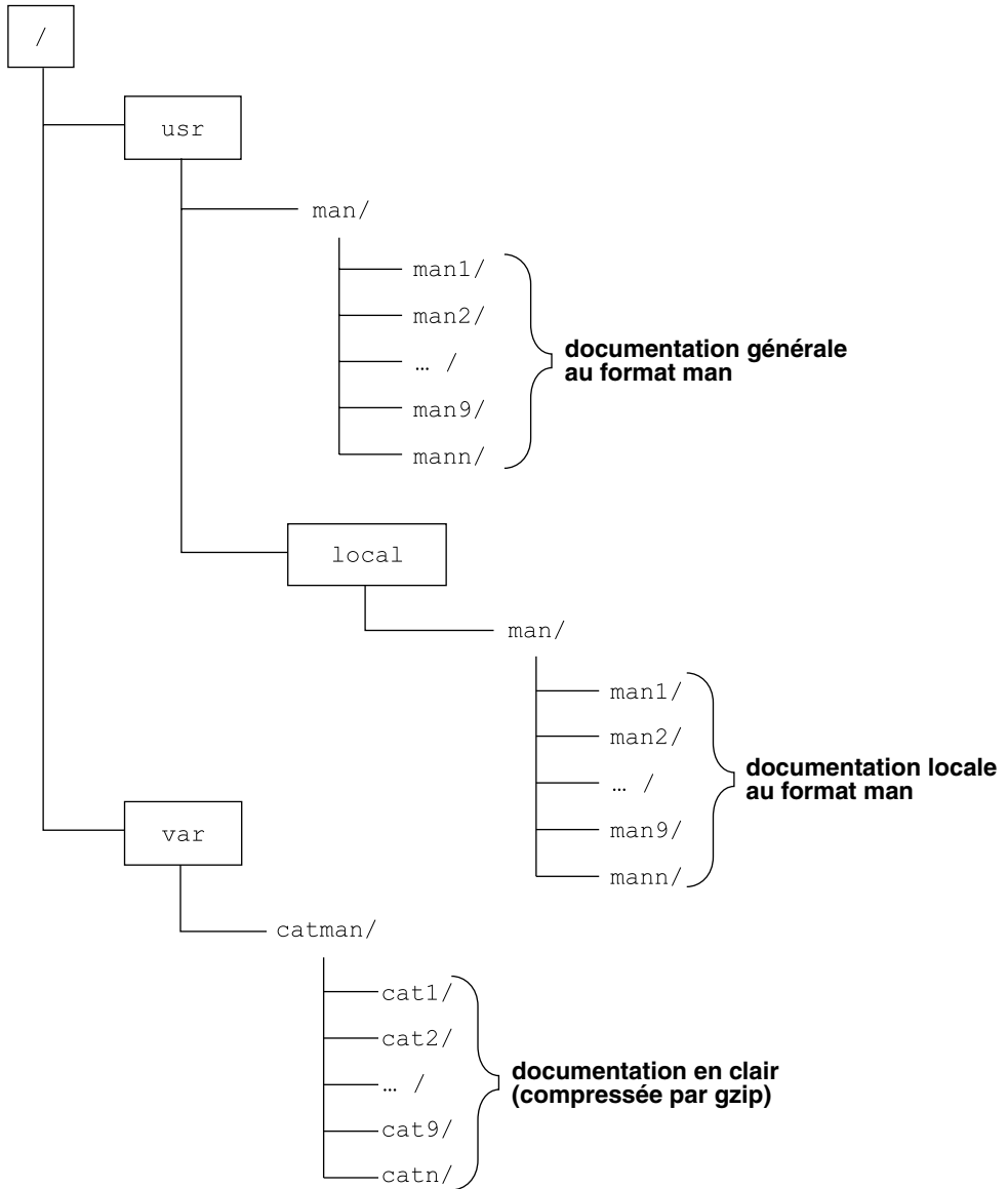
FIGURE 3.2. SOUS-ARBORESCENCE DU MANUEL.
