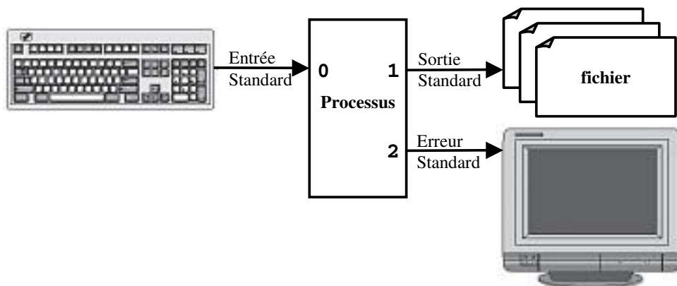
FIGURE 7.2. REDIRECTION VERS LE FICHIER FS DE LA SORTIE STANDARD D'UN PROCESSUS.
