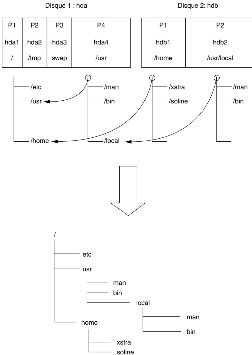
FIGURE 10.1. LES PARTITIONS ET L'ARBORESCENCE DES FICHIERS.
