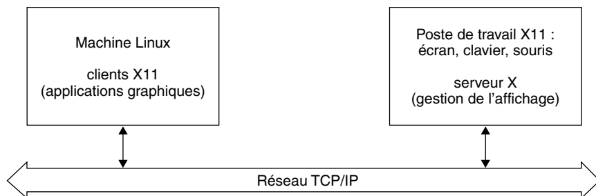
FIGURE 16.1. UN EXEMPLE D'UTILISATION DE X11 EN MODE CLIENT-SERVEUR : LE POSTE DE TRAVAIL ET LA MACHINE LINUX SONT DISTINCTS.
