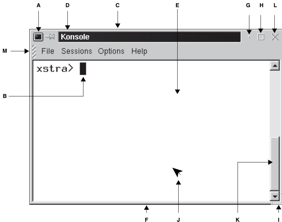
FIGURE 16.2. UNE FENÊTRE X11 SOUS LE GESTIONNAIRE DE FENÊTRE KWM.
