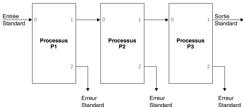
FIGURE 7.4. UN TUBE (PIPE).
