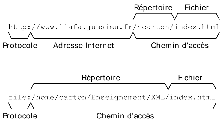
Figure 2.2. Structure d'une URL
