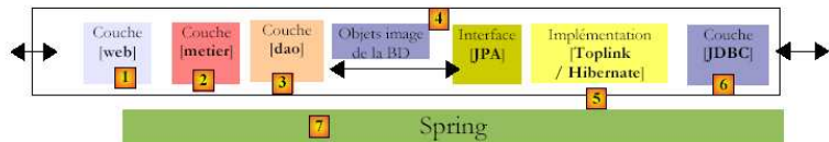
Fig.: Architecture multicouche avec JPA
