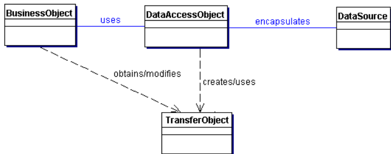
Fig.: Pattern DAO en Java
