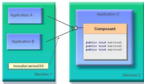
Principe des appels de procédure à distance
