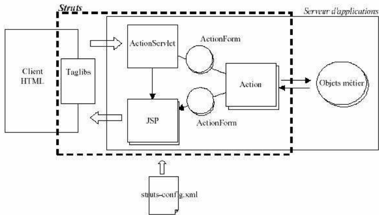
Fig.: Struts - détails
