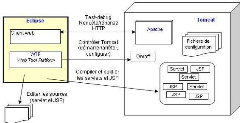
Fig.: Archi JSP/Tomcat
