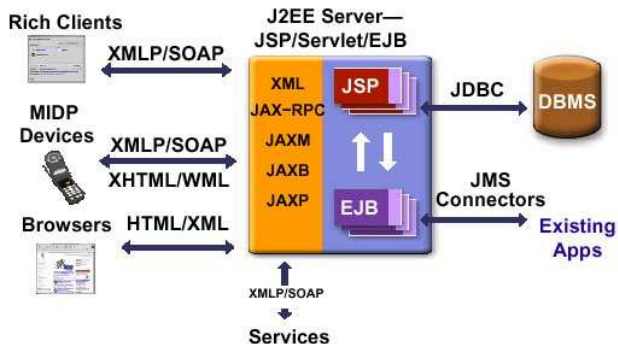
Fig.: Vision service Web
