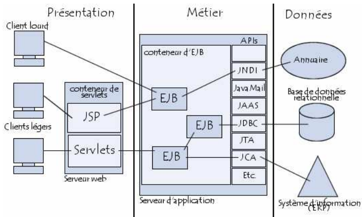
Fig.: Vue globale
