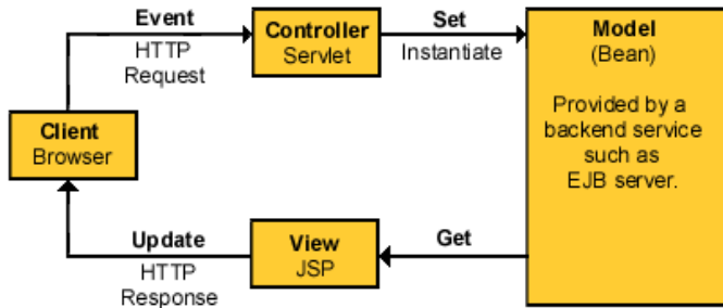
Fig.: Rôles dans Struts
