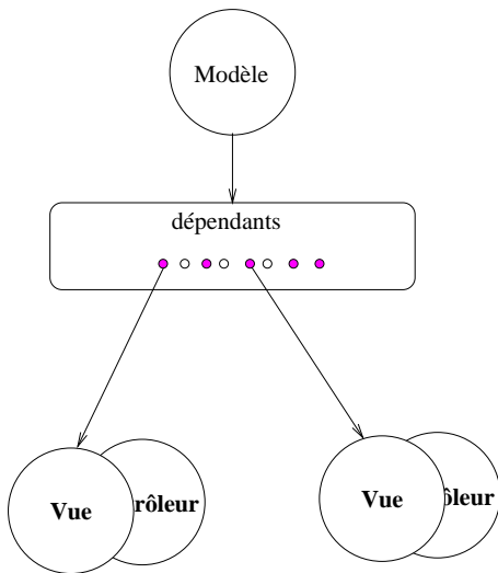
Fig.: MVC 4.0 Smalltalk
