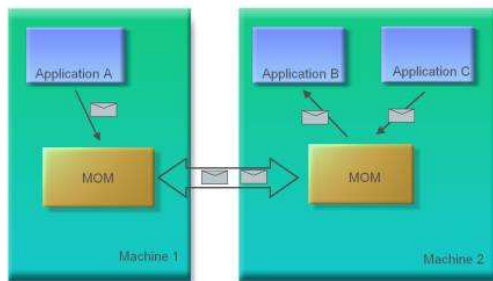
Principe des « Middleware Oriented Message »
