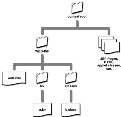
Fig.: Déploiement J2EE (varie selon le serveur)
