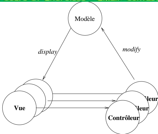
Fig.: MVC simplifié Smalltalk
