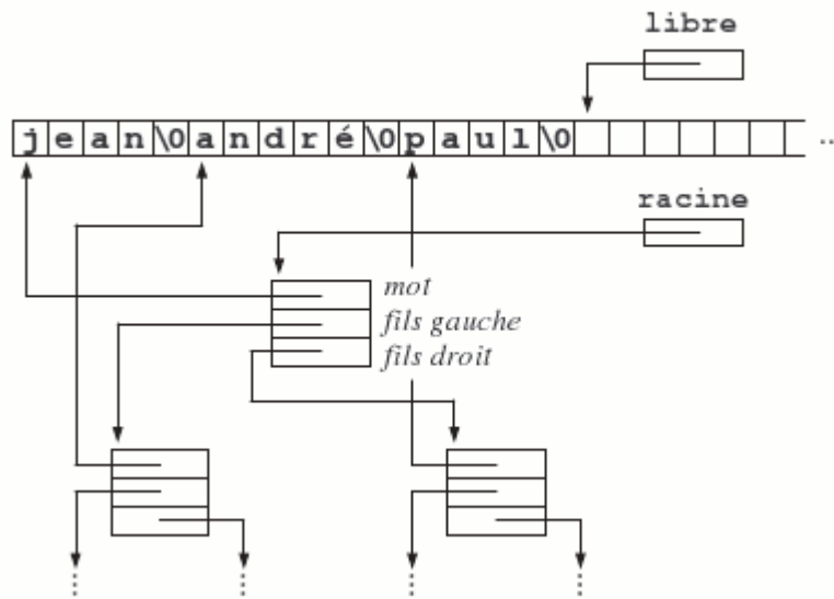
Fig. 16 - Arbre binaire de mots
