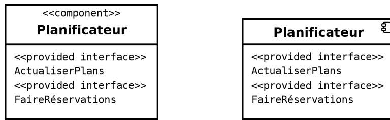
FIG. 8.1 – Représentation d’un composant et de ses interfaces requises ou offertes sous la forme d’un classeur structuré stéréotypé « component ». Au lieu ou en plus du mot clé, on peut faire figurer une icône de composant (petit rectangle équipé de deux rectangles plus petits dépassant sur son côté gauche) dans l’angle supérieur droit (comme sur la figure de droite).
