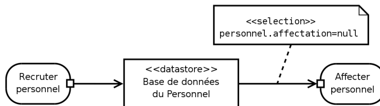
FIG. 6.10 – Dans cette modélisation, le personnel, après avoir été recruté par l'activité Recruter personnel , est stocké de manière persistante dans le nœud de stockage Base de donnée du Personnel . Bien qu'ils restent dans ce nœud, chaque employé qui n'a pas encore reçu d'affectation (étiquette stéréotypée «selection» : personnel.affectation=null ) est disponible pour être utilisé par l'activité Affecter personnel .
