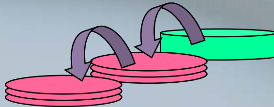
Volume fractionné
