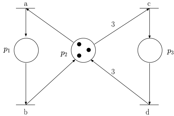
FIG. 3.1 – Exemple de réseau de Petri
