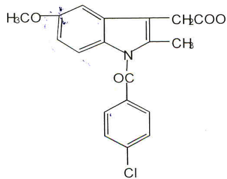
Indométacine
