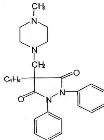
Pipébutazone
