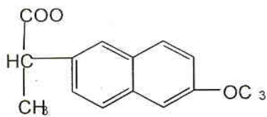
Naproxène
