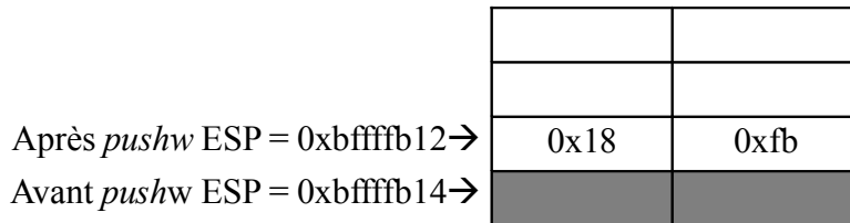
Figure 10 : Effet du pushw sur la pile
