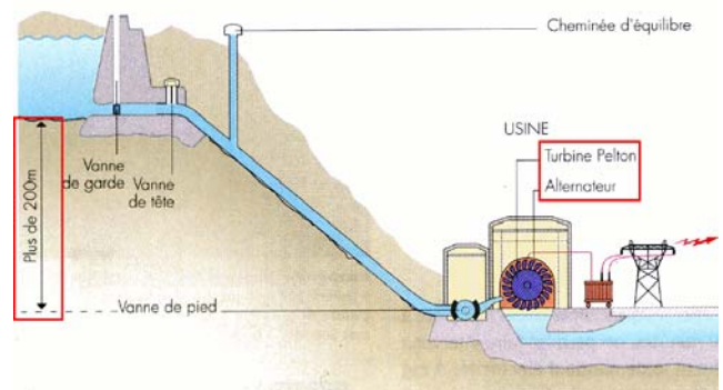
Fig-5a : Chute d'eau importante >200m de hauteur
