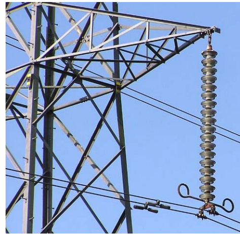
Figure 37 : Chaîne d'isolateurs sur un pylône de THT.
