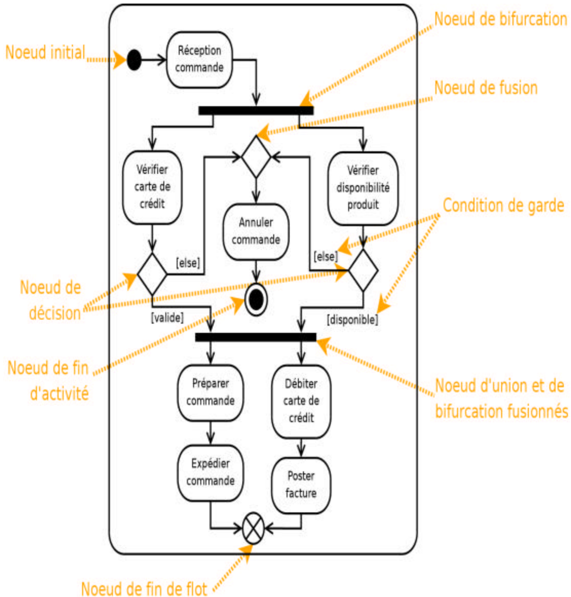
Diagramme d'activité illustrant l'utilisation de noeuds de contrôle. Ce diagramme décrit la prise en compte d'une commande.
