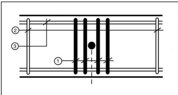
1 – Renforts adaptés. 2 – Etriers courants de chaînage de bord de dalle. 3 – Aciers filants de chaînage de bord de dalle.
