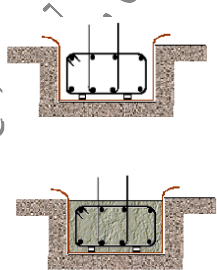
MISE en PLACE du FERRAILLAGE et BETONNAGE sans COFFRAGE
