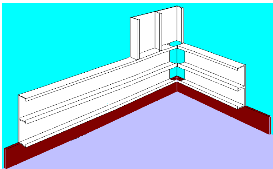
Figure 3-10 -Raccordement de moulures horizontales et verticales
