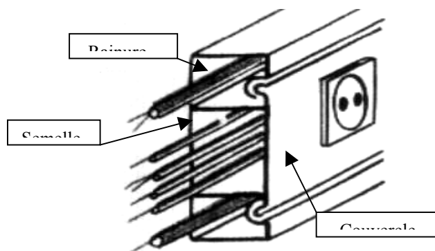
Goulotte a parois pleines
