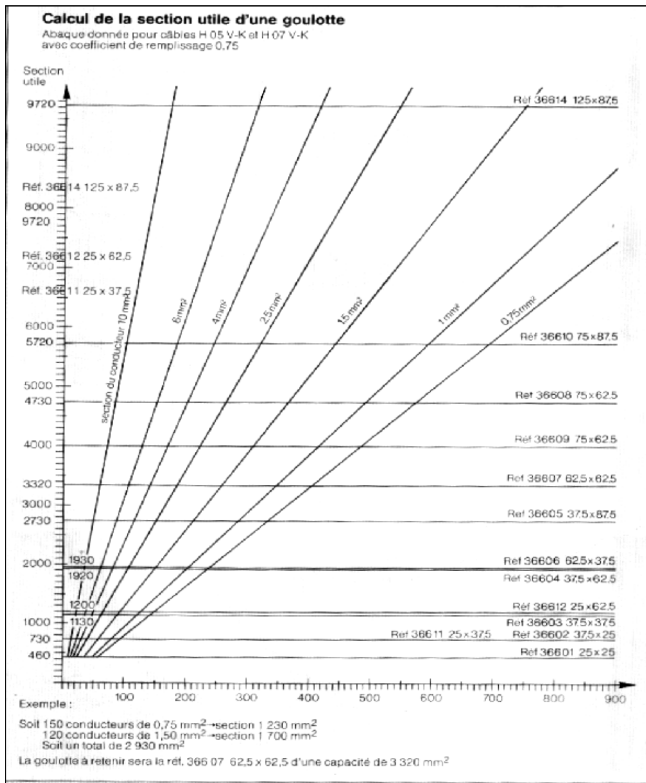
Figure 4-5 Goullotes Lina 25 à parois perforées (document LEGRAND)
