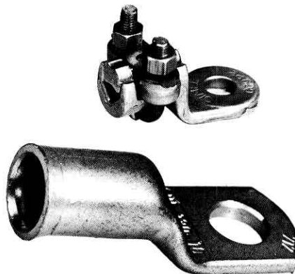
Figure 1-19 La cosse sertie écrase le conducteur en fil souple D'après Simel
