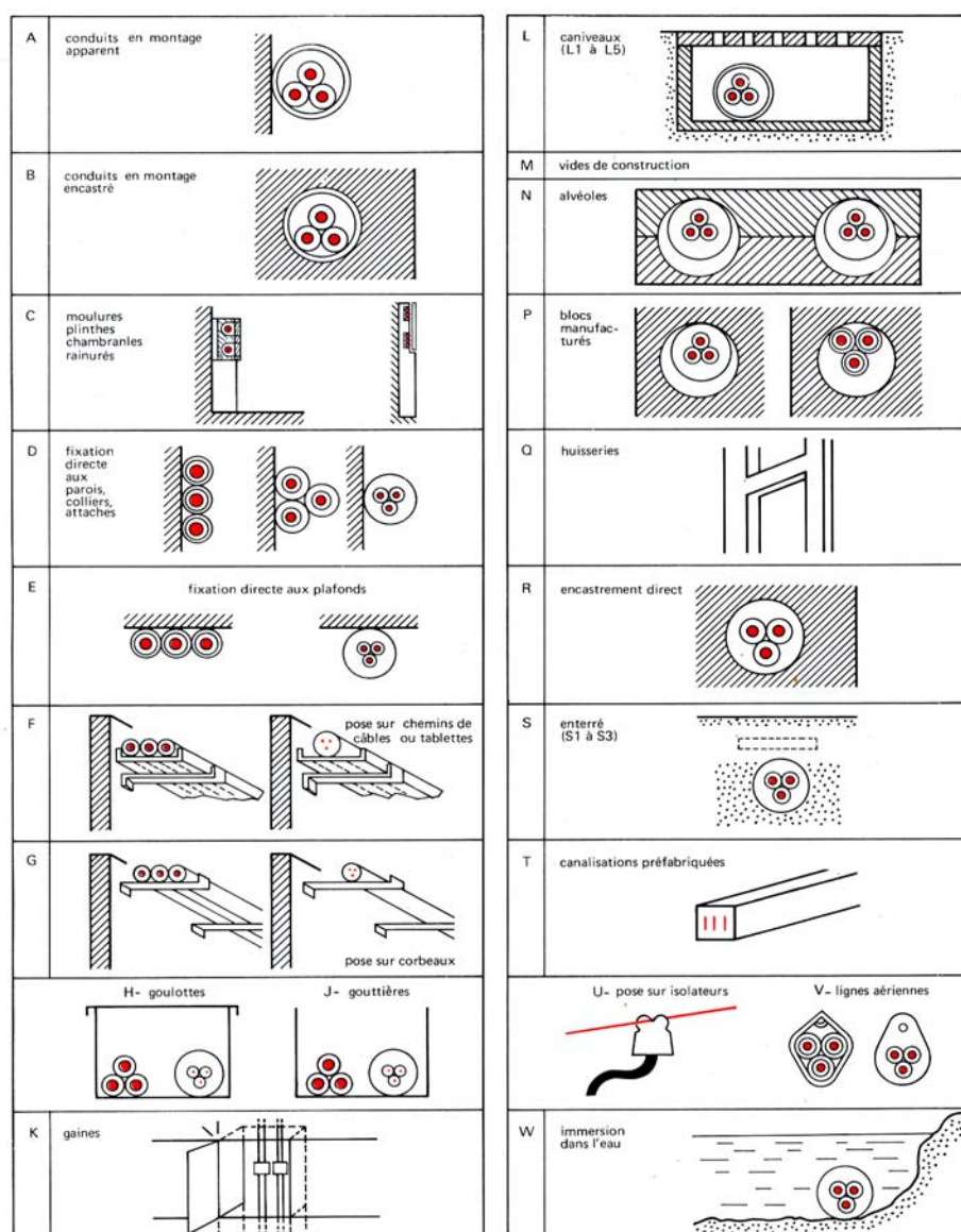
Figure 3-1- Tableau résumant les divers modes de poses des canalisations électriques
