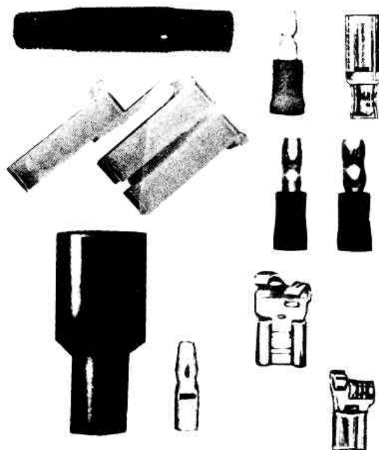
Figure 1-22 Connecteurs spéciaux à sertir
