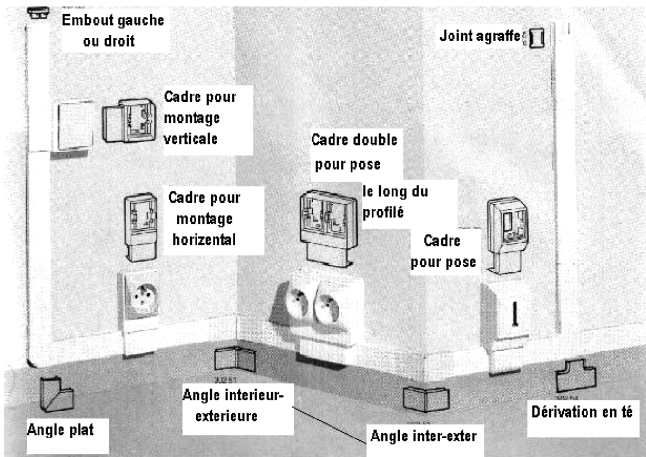
Figure 5-1 INSTALLATION DES MOULURES Moulure 32 x12,5
