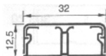
Avec cloison centrale
