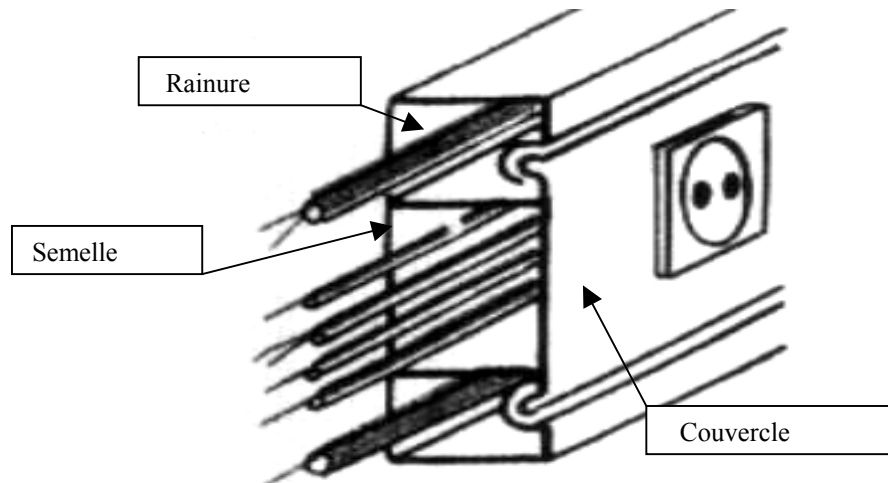
Goulotte à parois pleines
