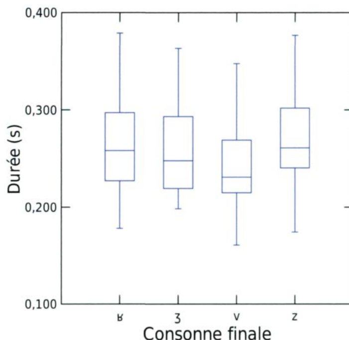
Figure 16 : Diagramme boîtes à moustaches présentant la durée des voyelles allongées en fonction de la consonne suivante.
