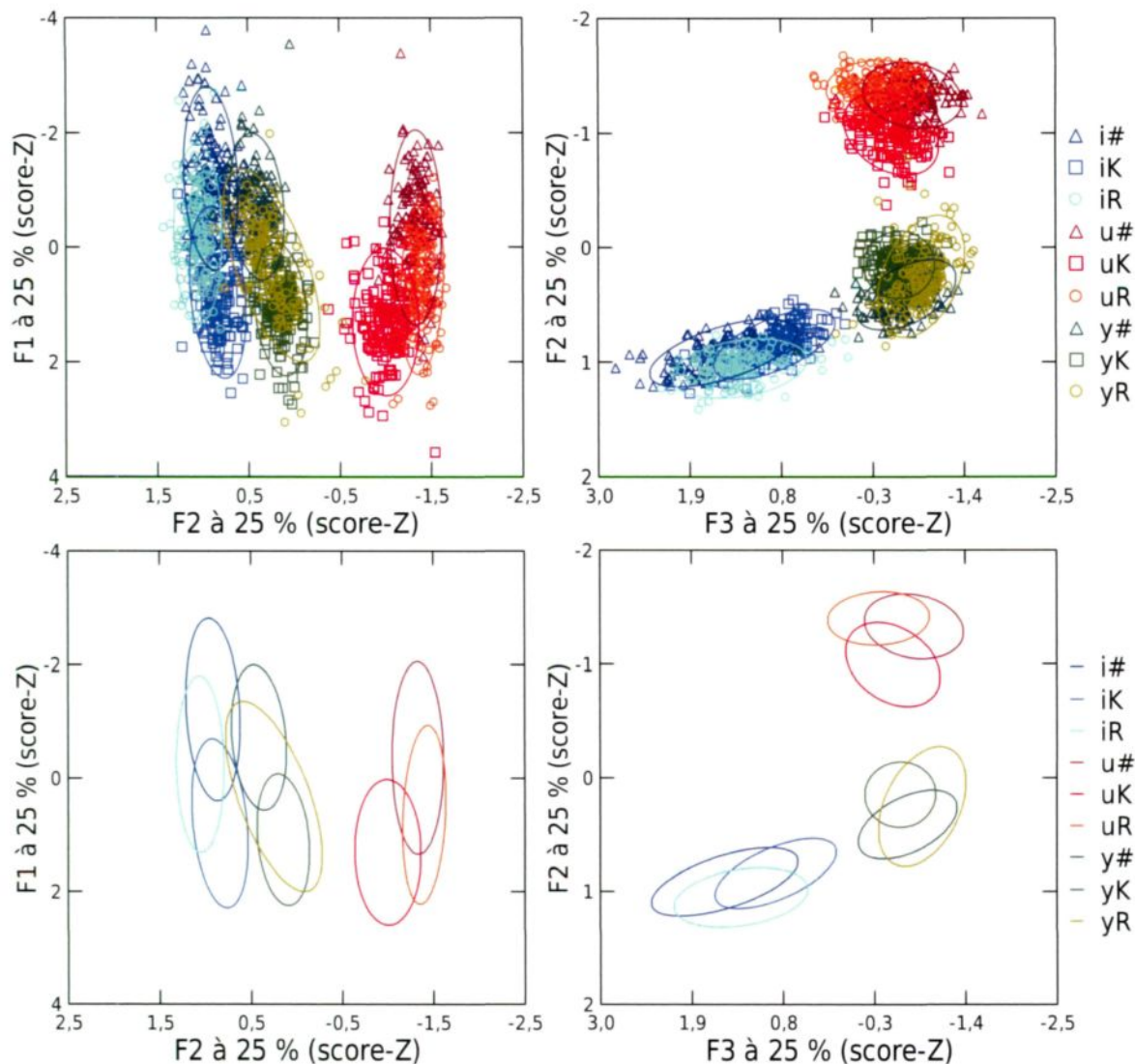
Figure 17 : Diagrammes bifurcés F_1 / F_2 et F_2 / F_3 normalisés présentant les 1343 occurrences analysées à 25 % de leur durée regroupées en fonction des classes vocaliques. Les ellipses de dispersion englobent 86,5 % des occurrences d'une même classe vocalique.
