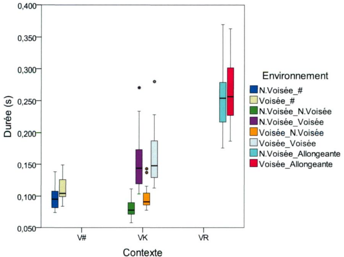
Figure 15 : Diagramme à boîtes à moustaches présentant la durée des variantes en fonction du contexte consonantique. Les astérisques indiquent des données extrêmes.
