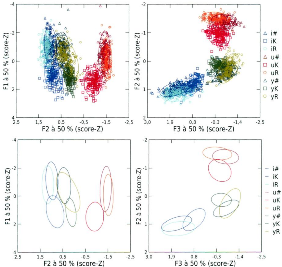
Figure 18 : Diagrammes bifurmantiques F_1 / F_2 et F_2 / F_3 normalisés présentant les 1343 occurrences analysées à 50 % de leur durée regroupées en fonction des classes vocaliques. Les ellipses de dispersion englobent 96,5 % des occurrences d'une même classe vocalique.
