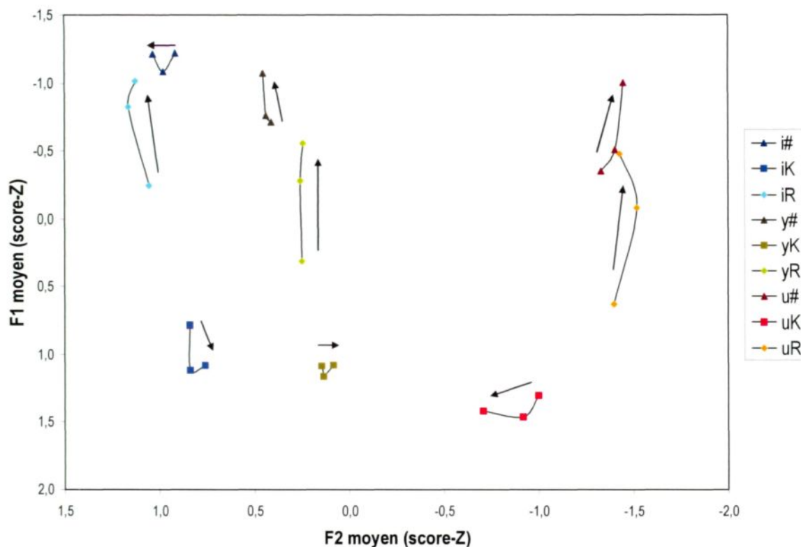
Figure 24 : Diagramme bifurmantique F_1 / F_2 normalisés présentant l'évolution moyenne des différentes classes vocales, tous locuteurs confondus.
