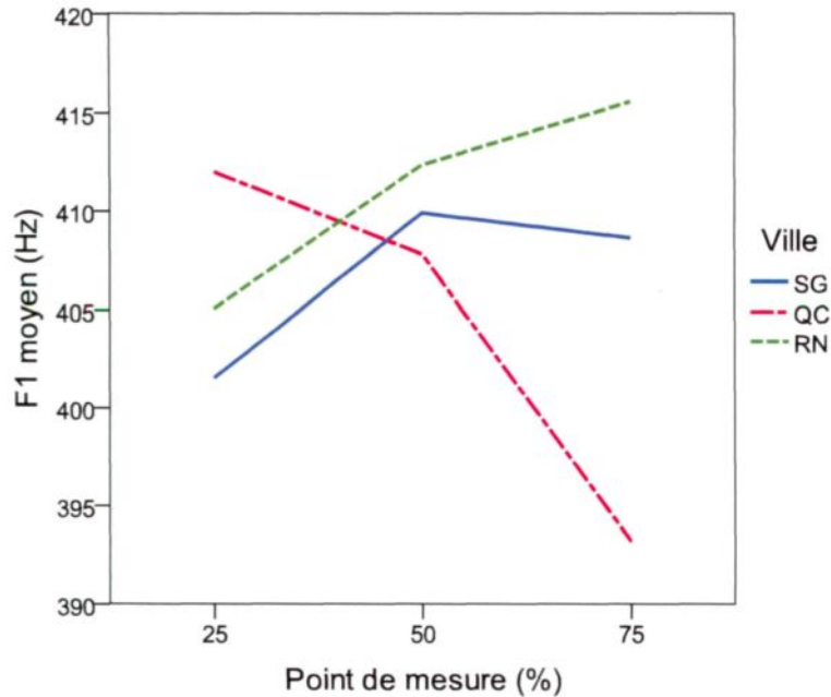
Figure 23 : Trajectoire temporelle moyenne du F 1 de la classe vocalique (yK) en fonction de la ville d'origine des locuteurs.
