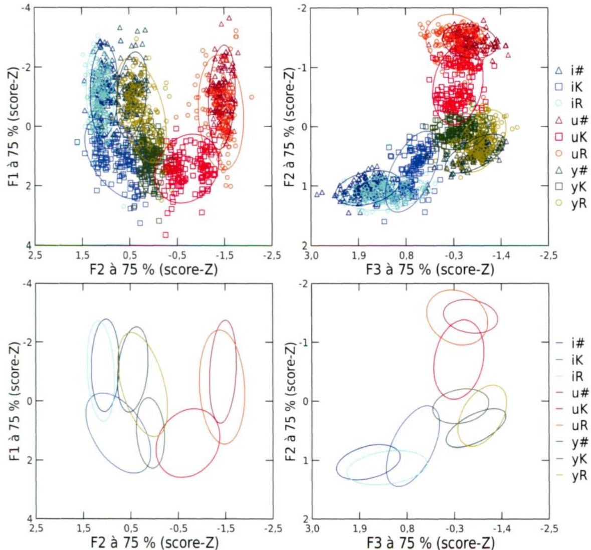
Figure 19 : Diagrammes bifurmantiques F_1 / F_2 et F_2 / F_3 normalisés présentant les 1343 occurrences analysées à 75 % de leur durée regroupées en fonction des classes vocaliques. Les ellipses de dispersion englobent 86,5 % des occurrences d'une même classe vocalique.
