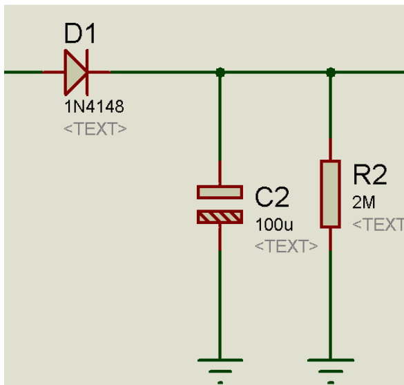
Figure III.18 : Détecteur d'enveloppe.
