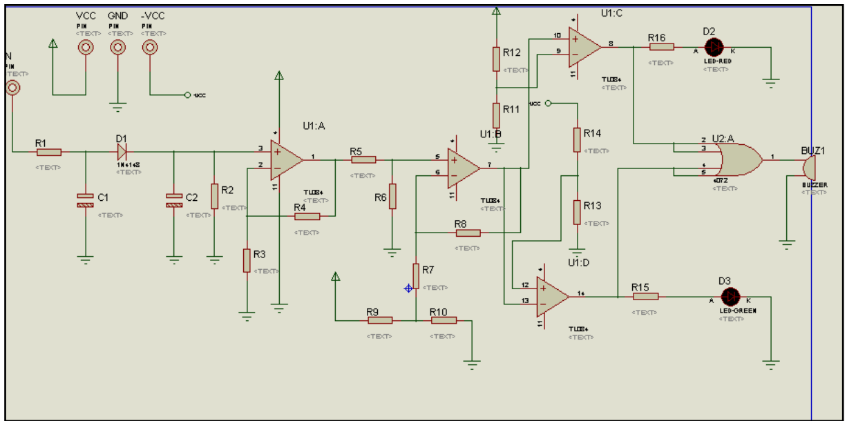
Figure II.19 : Circuit d'alarme
