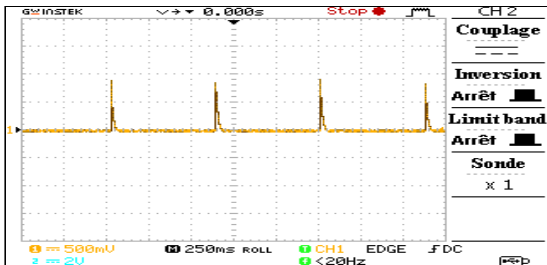
Figure III.7 : Signal de sortie du générateur d'impulsions (unidirectionnel).
