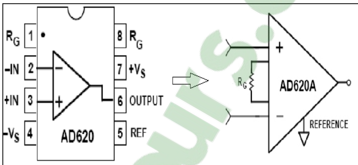
Amplificateur d'instrumentation AD620
