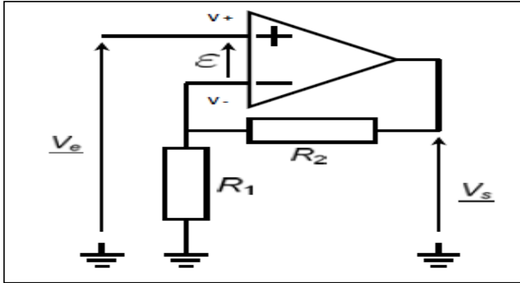
Figure II.23 : Ampli non-inverseur
