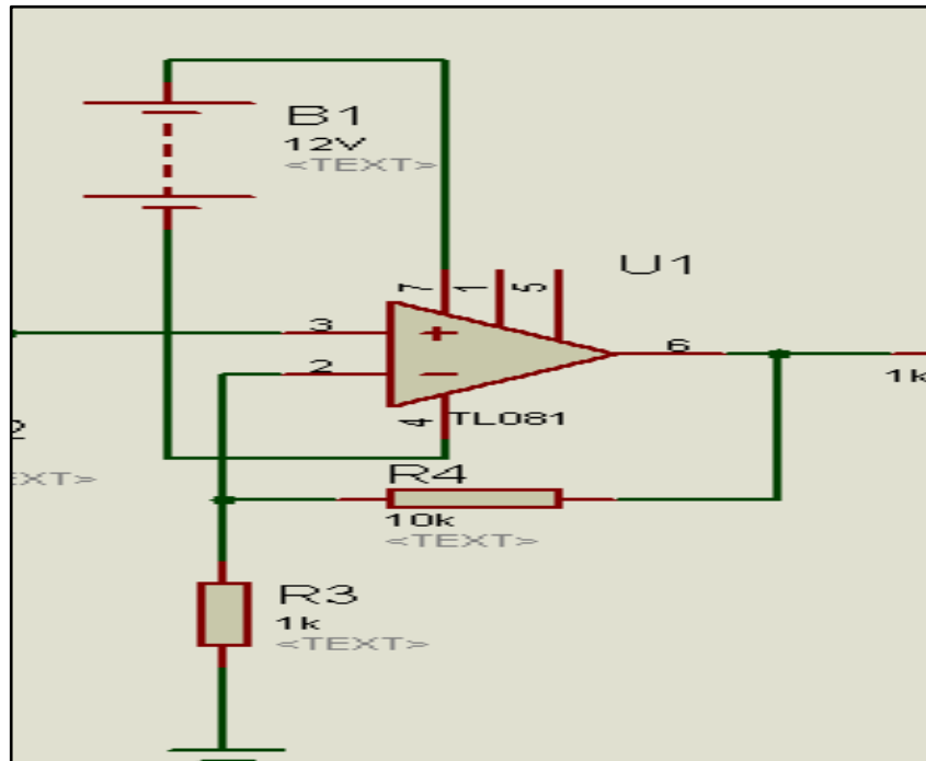
Figure III.20 : Amplificateur non-inverseur
