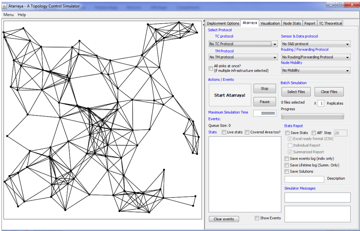
Figure IV.6: La fenêtre de l'onglette Atarraya.
