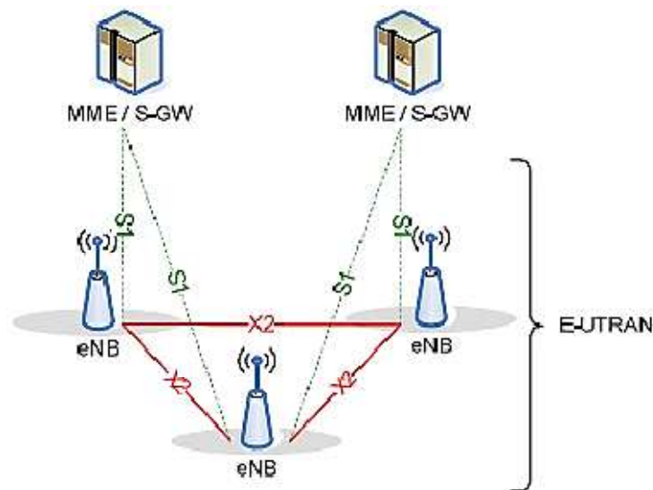
Figure II.3 : Les interfaces existant dans l'E-UTRAN.
